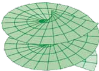
Fig. Helicoide
